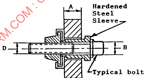
FIGURE D1 - TORQUE OUT TEST APPARATUS
