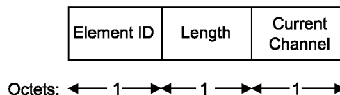
Figure 38—DS Parameter Set element format
