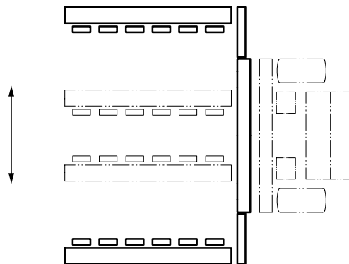
Figure 16 — Brick clamp Figure 16 — Pince à briques
