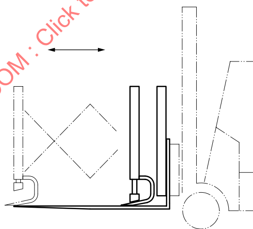
Figure 26 — Push/pull attachment Figure 26 — Pousseur/tireur de charge
