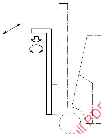
Figure 38 — Telescopic side lift spreader Figure 38 — Spreader télescopique à prise latérale
