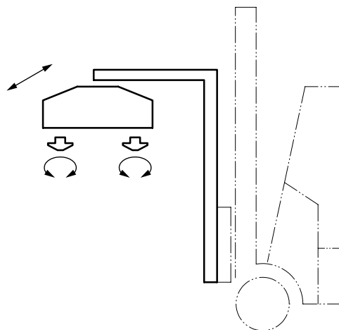
Figure 36 — Telescopic spreader Figure 36 — Spreadre télescopique
