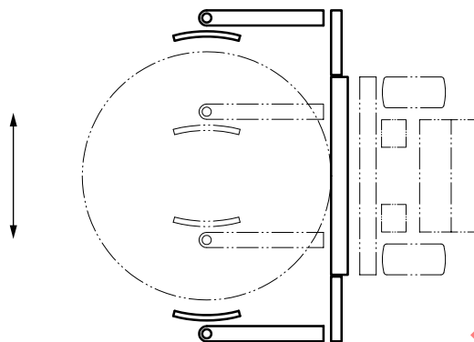
Figure 20 — Roll clamp Figure 20 — Pince à rouleau
