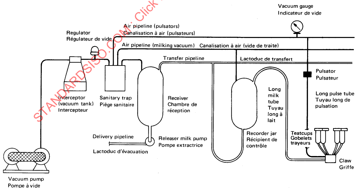
FIGURE 3 — Machine à traire avec lactoduc de traite
