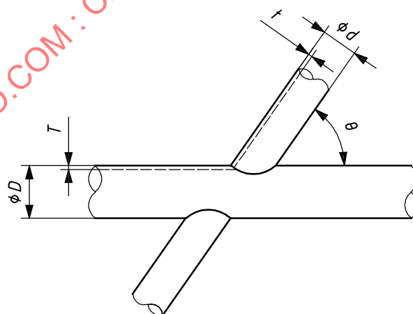
b) X-joint
