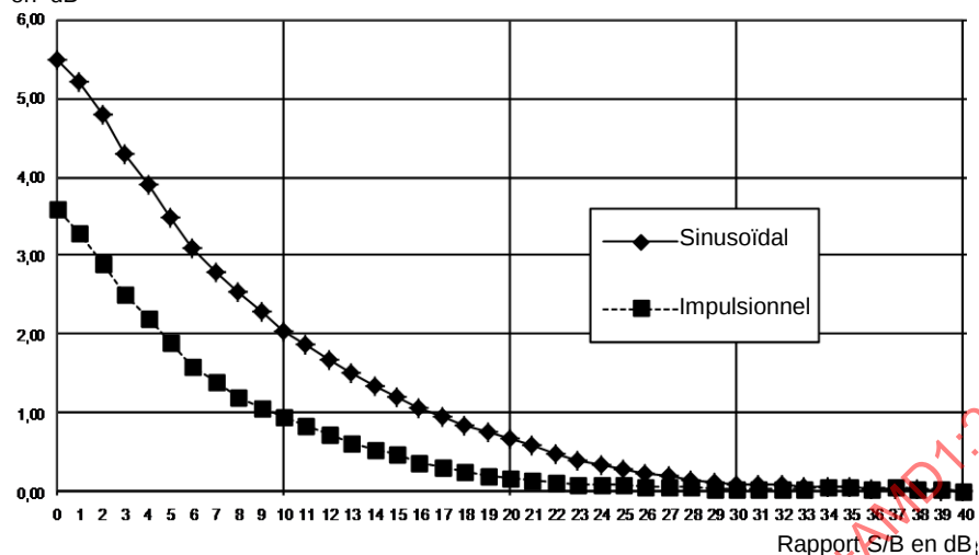
Figure A.2 – Écart de l'indication de niveau du détecteur de crête par rapport au niveau du signal à l'entrée du récepteur, pour deux cas: signal sinusoïdal et signal impulsionnel (PRF de 100 Hz)
