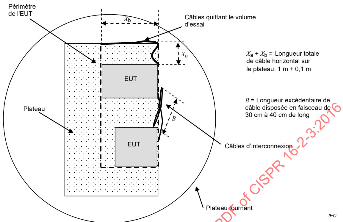
Figure 17 – Installation d'essai pour un matériel posé sur table – Vue de dessus
