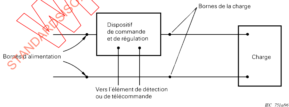
Figure 12a – Disposition dans le cas de la mesure d'un dispositif de commande et de régulation à deux bornes
