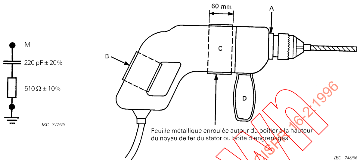
Figure 8 – Élément RC pour main artificielle (voir 2.4.4.2.3)
