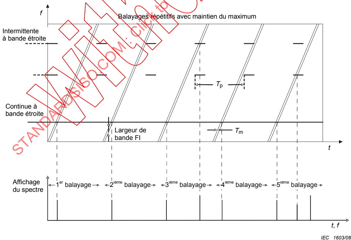
Figure 5 – Perturbations intermittentes à bande étroite mesurées en utilisant des balayages courts, rapides et répétitifs avec la fonction «maintien du maximum» pour obtenir une vue d'ensemble du spectre d'émission
