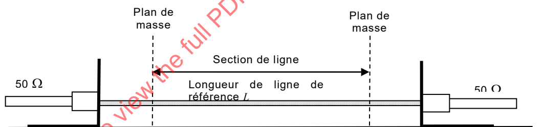
Figure 27d – Configuration pour la mesure d'étalonnage "ligne"
