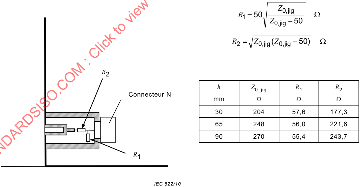
Figure 31 – Exemple d'adaptateur avec réseau d'adaptation résistif
