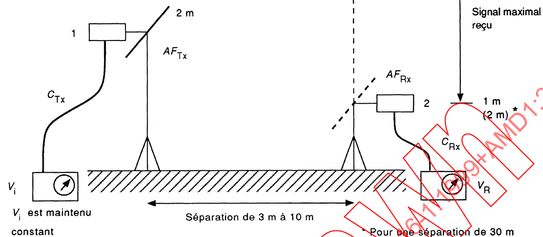
Figure 16 – Configuration des équipements pour la mesure en polarisation horizontale de l'affaiblissement de l'emplacement. Voir 5.6.6 et annexe G pour plus de détails
