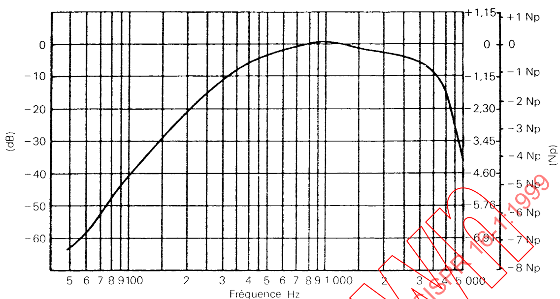
Figure 5 – Courbe caractéristique du réseau filtrant psophométrique utilisé pour les mesures aux bornes d'un circuit téléphonique commercial interurbain (voir 4.6.1.3, point b))
