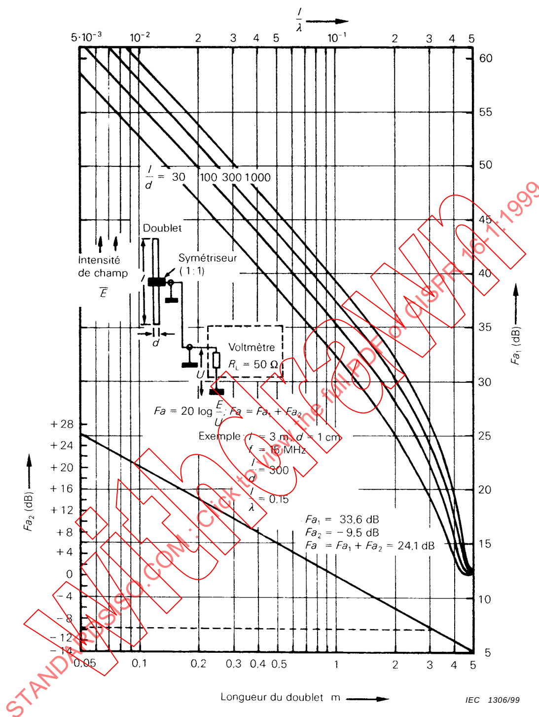
Figure 13 – Facteurs d'antenne des doublets courts pour R_L = 50 \Omega (voir 5.5.4.1.2)
