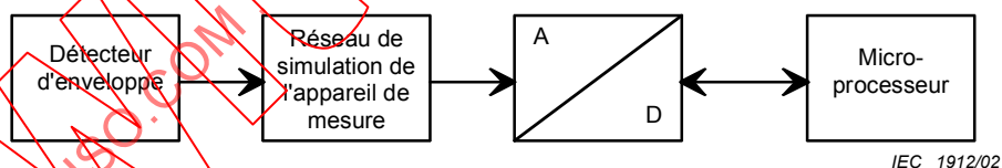
Figure 5 – Schéma fonctionnel d'un détecteur de valeur moyenne
