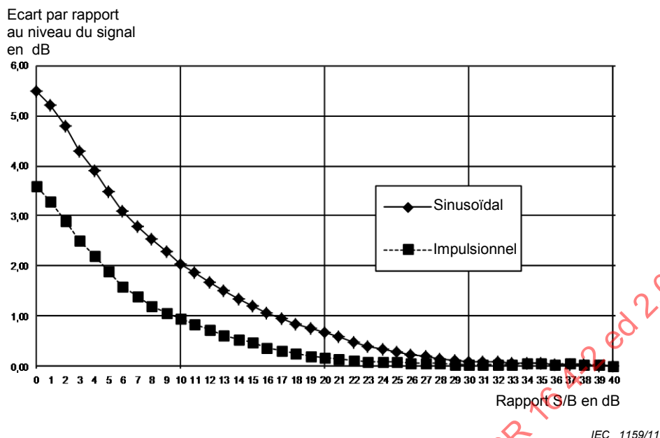
Figure A.2 – Écart de l'indication de niveau du détecteur de crête par rapport au niveau du signal à l'entrée du récepteur, pour deux cas: signal sinusoïdal et signal impulsionnel (PRF de 100 Hz)
