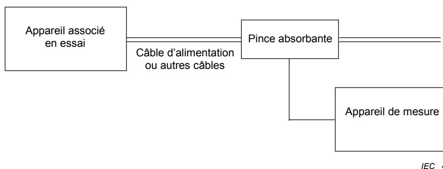
Figure 10 – Disposition de mesure de la puissance perturbatrice des équipements associés (à l'exclusion des magnétoscopes) (voir 5.6.3)
