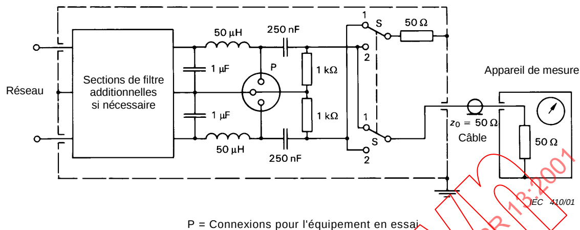
Figure 3 – Exemple d'un réseau fictif d'alimentation 50 Ω-50 μH (voir 5.3.1)
