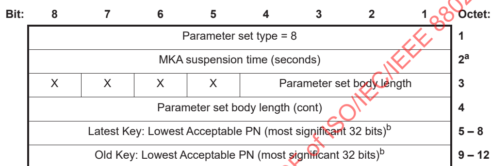
Figure 11-16—XPN parameter set
