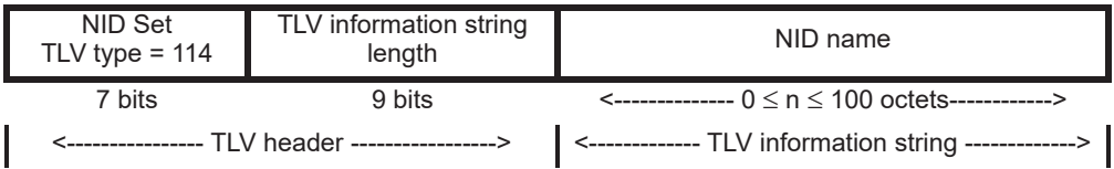
Figure 11-20—NID Set TLV format
