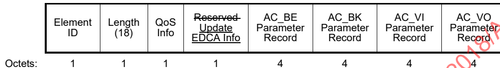
Figure 9-261—EDCA Parameter Set element
