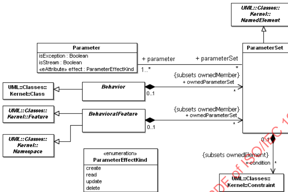
Figure 12.18 - Parameter sets
