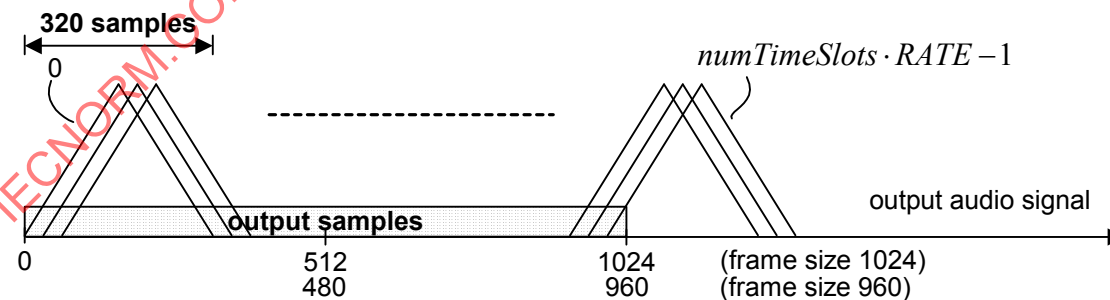
(d) output signal downsampled QMF synthesis windowing
