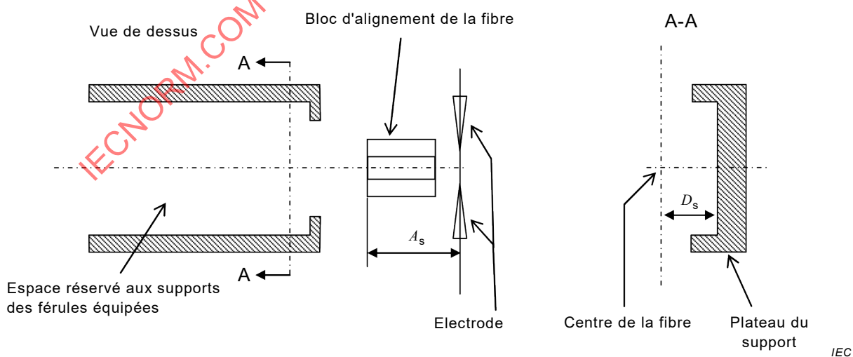
Figure 2 – Interface de l'épissureur par fusion
