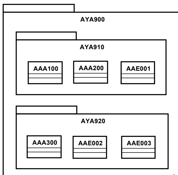
Figure 19 – Diagramme de paquetage UML par relations
