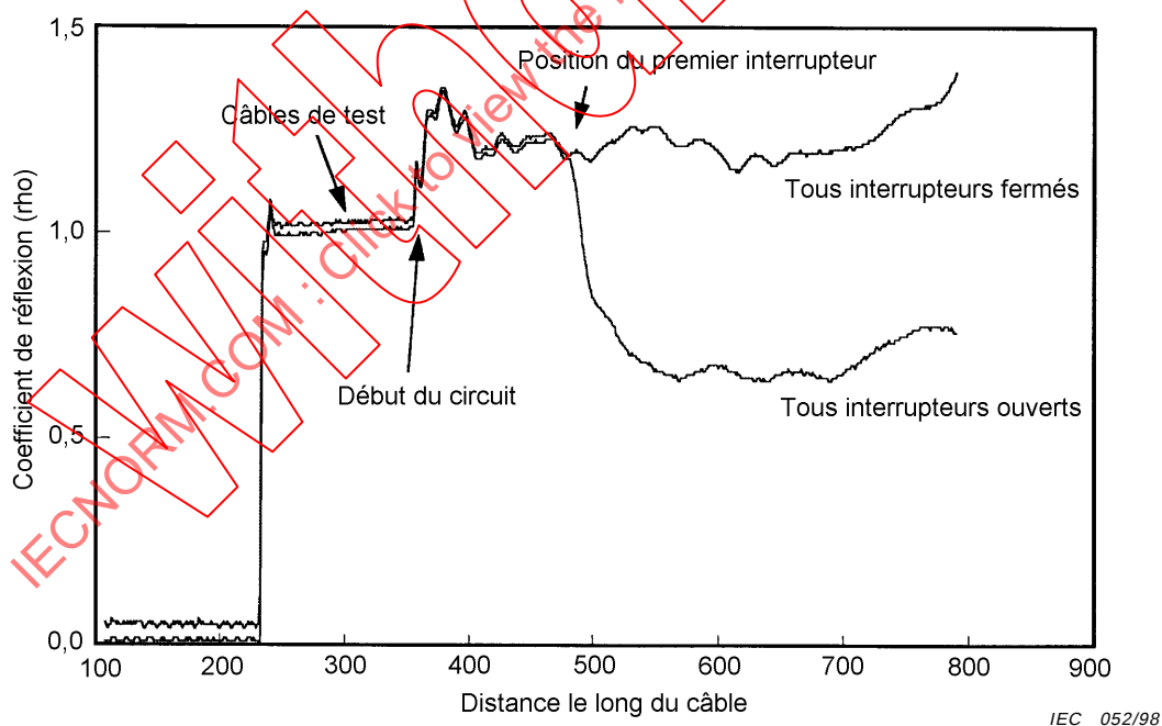
Figure 21 – Profil des spectres du domaine temporel pour un circuit d'éclairage avec interrupteurs ouverts et fermés, montrant l'emplacement du premier interrupteur
