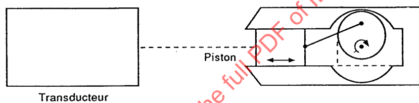
Figure 2 - Diagramme schématique d'un montage pour essai Doppler à bande, à disque et à piston
