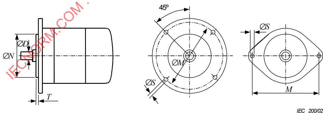
Figure 2 – Dimensions de montage des moteurs pas à pas à pôles à griffes
