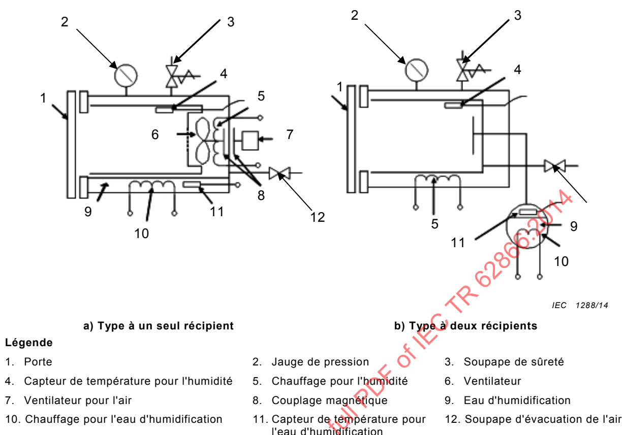
Figure 17 – Deux types de matériel d'essai HAST et leurs structures
