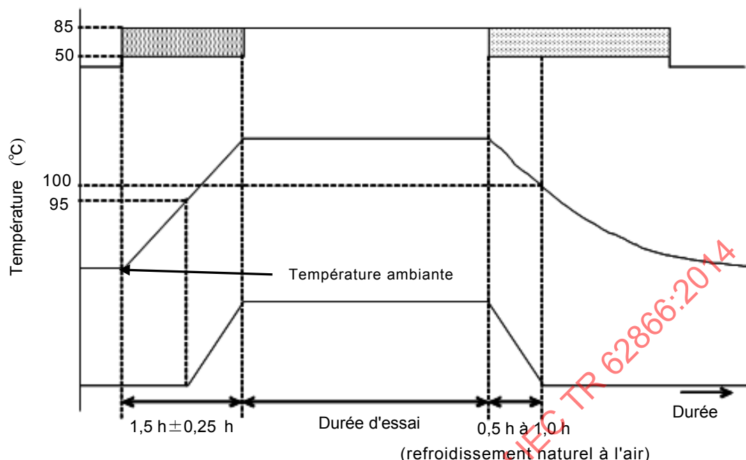
Figure 16 – Profil d'essai HAST
