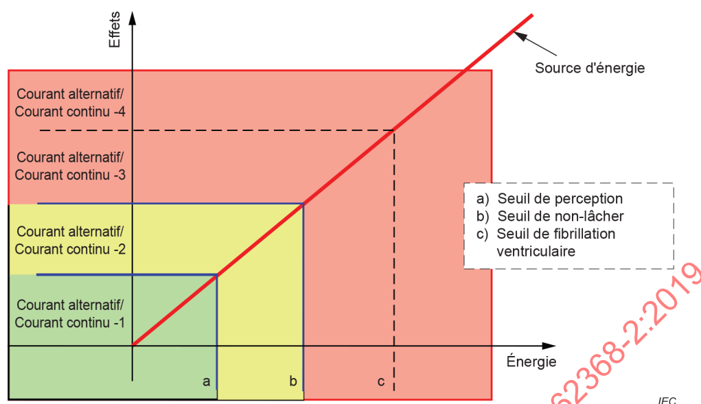
Figure 10 – Démonstration que les limites dépendent de la tension et du courant
