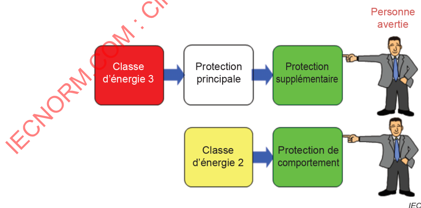
Figure 5 – Protections destinées à protéger une personne avertie
