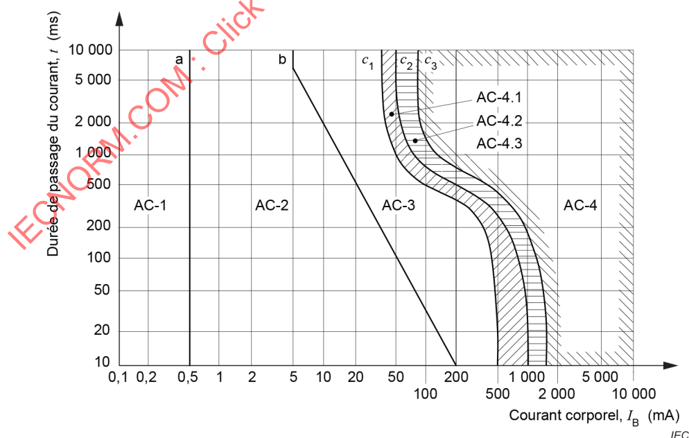
Figure 8 – Zones temps/courant conventionnelles des effets des courants alternatifs (15 Hz à 100 Hz) sur les personnes pour un trajet correspondant main gauche à pieds (voir l'IEC TS 60479-1:2005, Figure 20)
