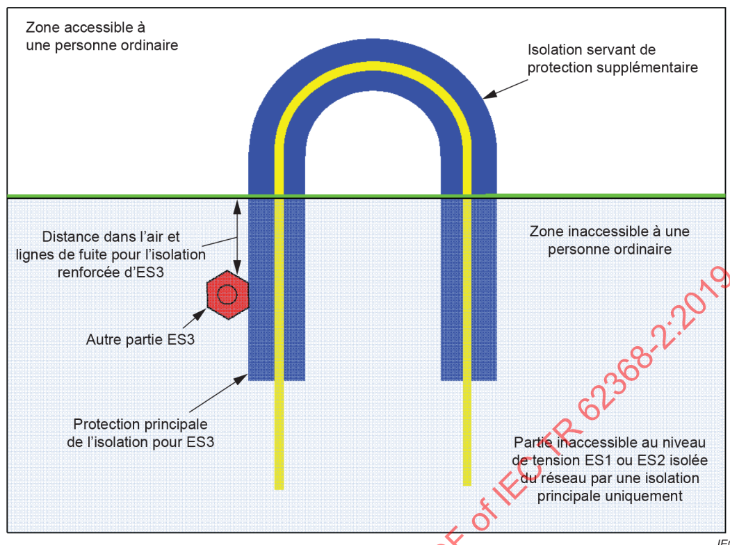
Figure 16 – Exemple illustrant le câblage interne accessible
