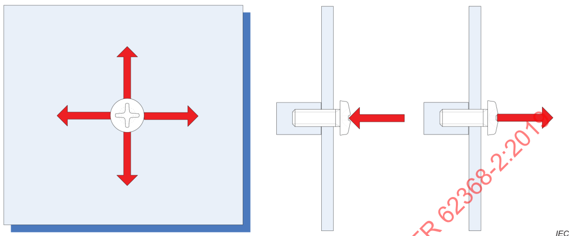
Figure 37 – Direction des forces à appliquer
