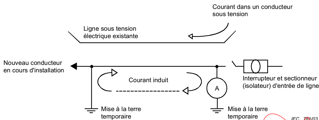
Figure 3a – Deux mises à la terre sur un nouveau conducteur permettent la circulation du courant
