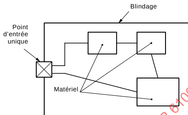
Figure 3a – Système de câblage maillé
