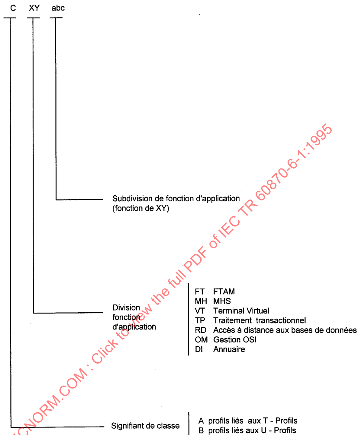
Figure B.2 – Structure d'un identifiant d'application
