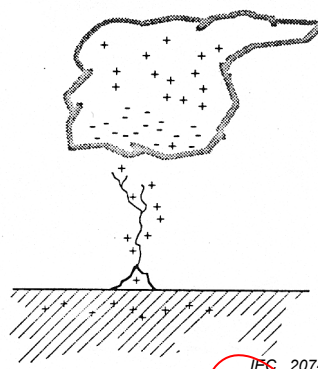
Figure 1b – La foudre comporte un traceur chargé positivement et donc, ce type diminue réellement la charge négative du sol
