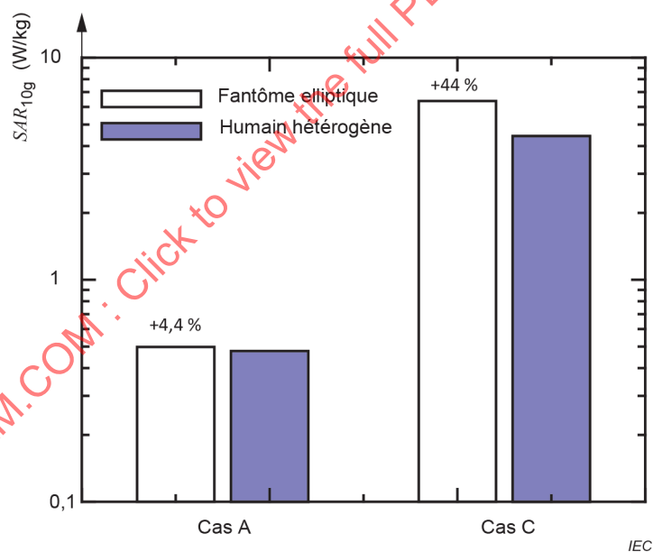
Figure D.5 – DAS calculé pour les petites bobines carrées de 10 cm × 10 cm qui fonctionnent à 2 cm du fantôme elliptique et du modèle humain hétérogène
