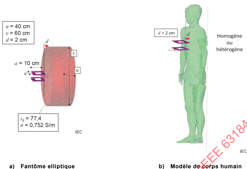
Figure D.4 – Modèle de simulation d'un système WPT de faibles dimensions qui fonctionne à proximité a) d'un fantôme elliptique et b) d'un modèle de corps humain
