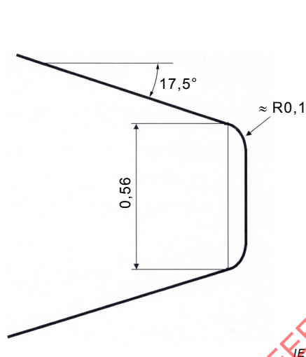
Figure 1 – Géométrie et dimensions correspondant au profil de l'extrémité de la sonde (cône tronqué) utilisée pour le poinçonnement
