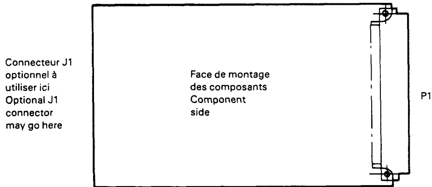
Fig. 3. - Désignation de référence de l'Eurocard. Eurocard reference designation.
