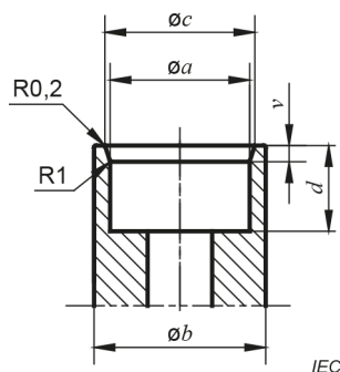
Figure 6 – Calibre pour un contact extérieur mâle
