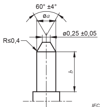
Figure 5 – Calibre pour un contact femelle de canal RF
