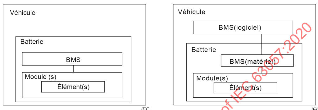
a) Toutes les fonctions du BMS se trouvent dans la batterie
