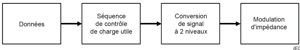
Figure 13 – Modulation et codage de la charge utile en liaison ascendante
