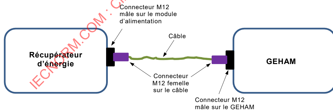
Figure A.2 – Option 2: Connecteurs reliés au récupérateur d'énergie et au GEHAM
