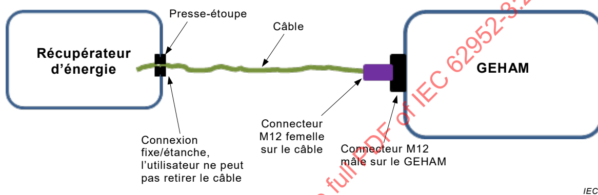
Figure A.1 – Option 1: Connexion fixe à un récupérateur d'énergie, connecteur relié au GEHAM
