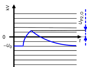
LCC ou VSC, tension de choc de manœuvre positive de polarité opposée
