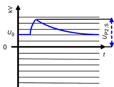
VSC, tension de choc de manœuvre positive de même polarité
