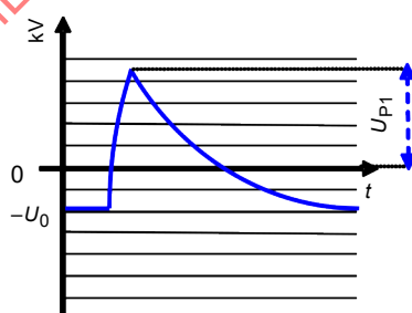
LCC ou VSC, tension de choc de foudre positive
