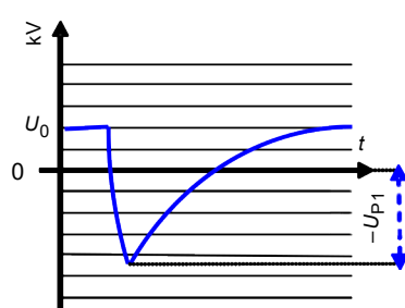
LCC ou VSC, tension de choc de foudre négative
