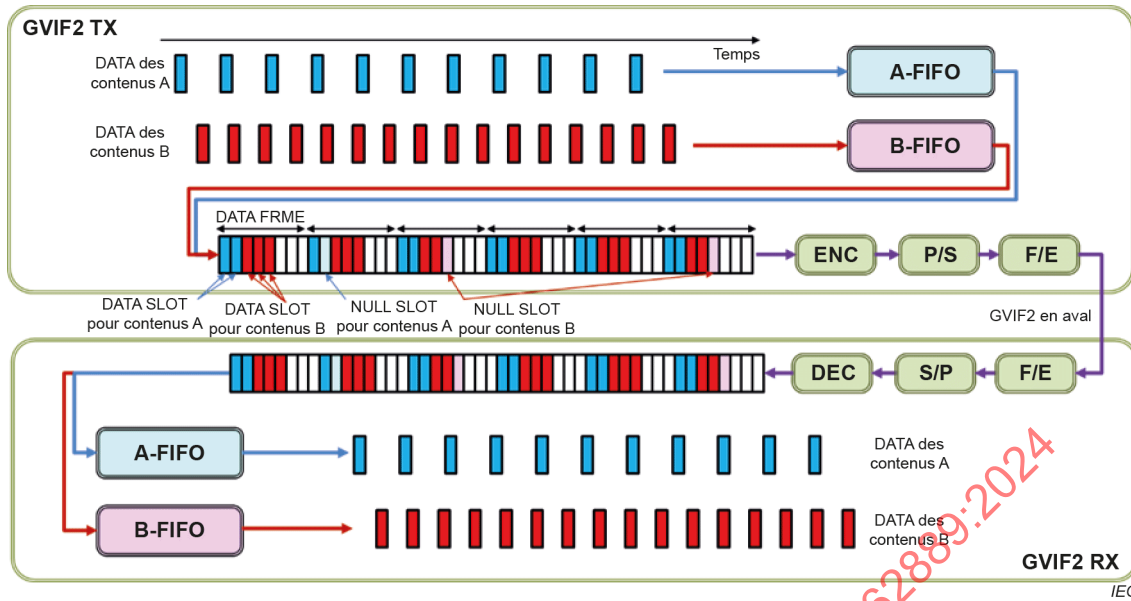
Figure A.2 – Transmission en multiplexe de la GVIF2 pour contenus multiples
