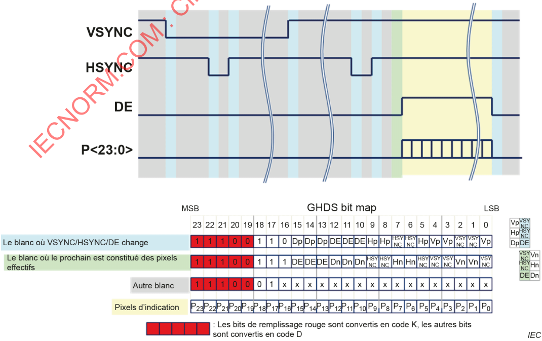
Figure 7 – Mappage des données RGB888 de la GVIF2
