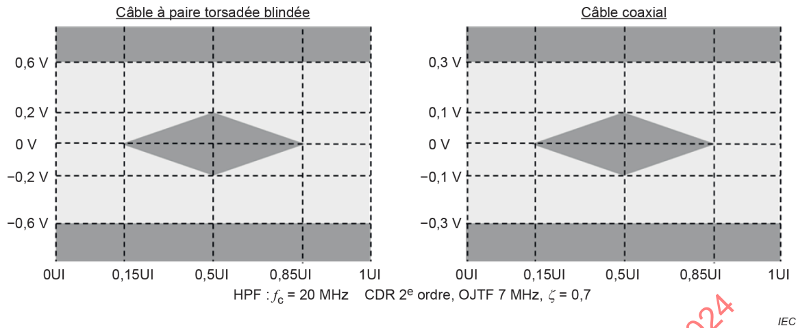
Figure 3 – Masque de l'œil en aval de la GVIF2 (au TP1)
