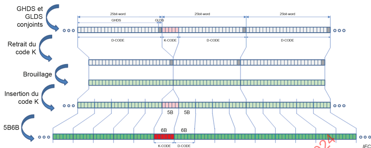
Figure 12 – Codage en aval
