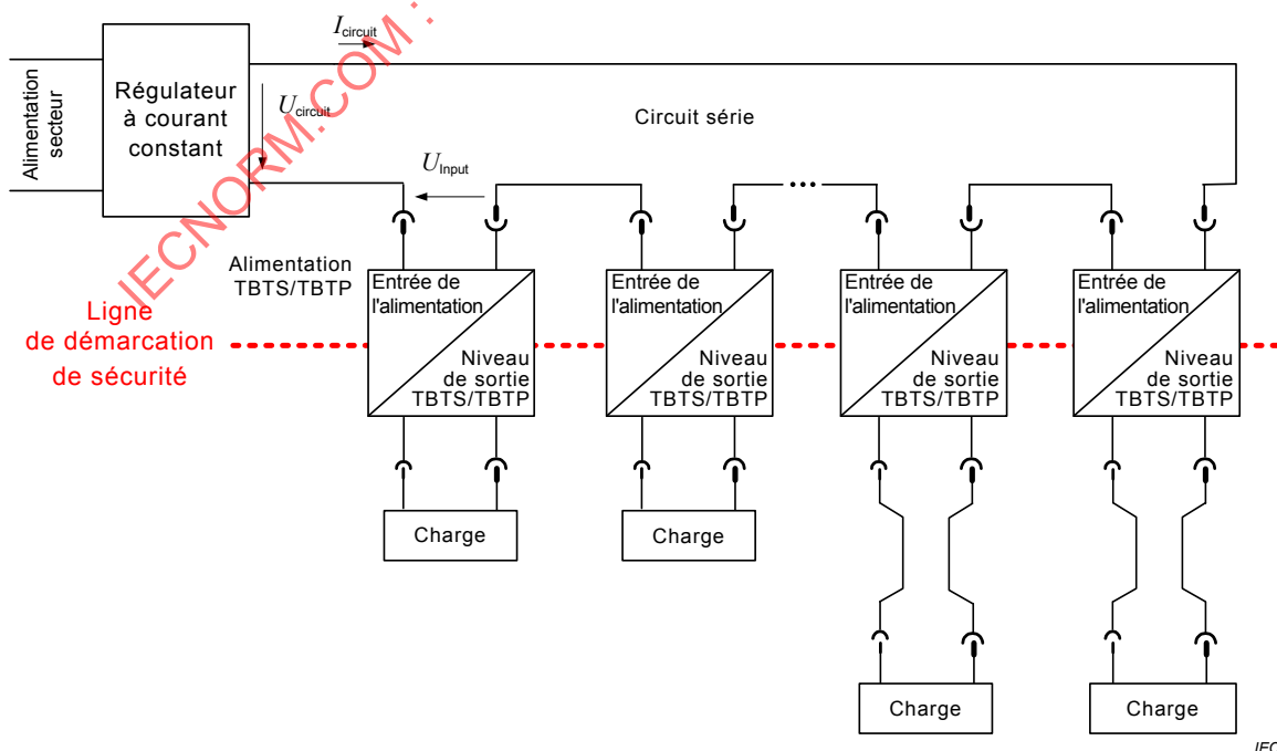
Figure 1 – Ligne de démarcation de sécurité dans un système TBTS
