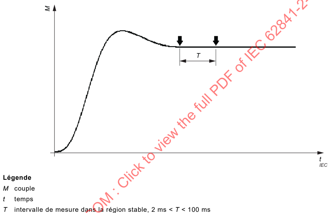
Figure 109 – Exemple de couple d'un outil avec région de signal stable
