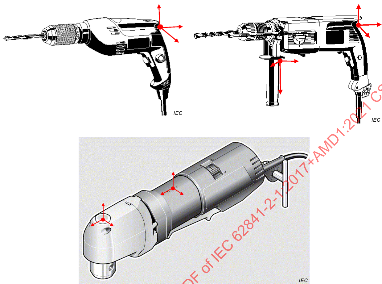
Figure I.102 – Positions des transducteurs pour les perceuses et les perceuses à percussion
