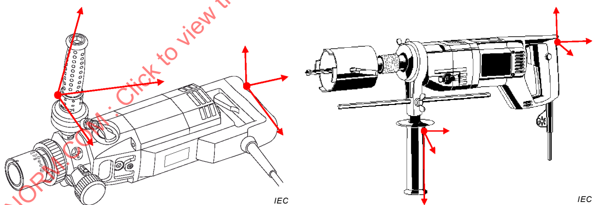
Figure I.103 – Positions des transducteurs pour les perceuses à diamant
