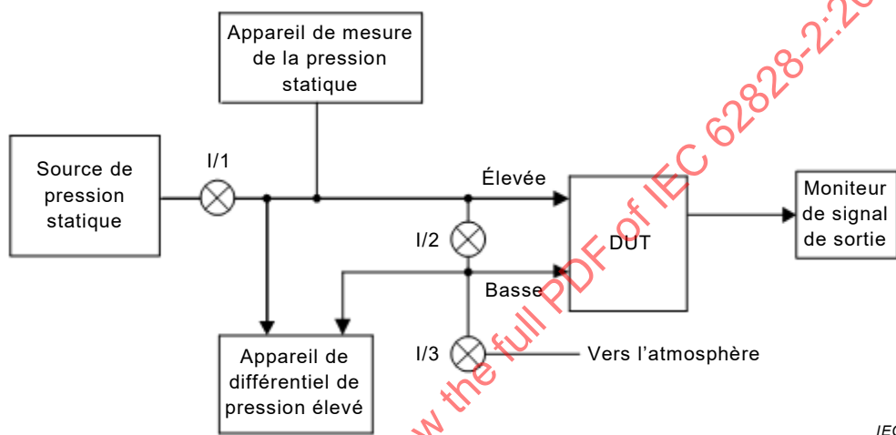
Figure 5 – Exemple schématique de montage d'essai permettant de déterminer l'effet de la pression statique
