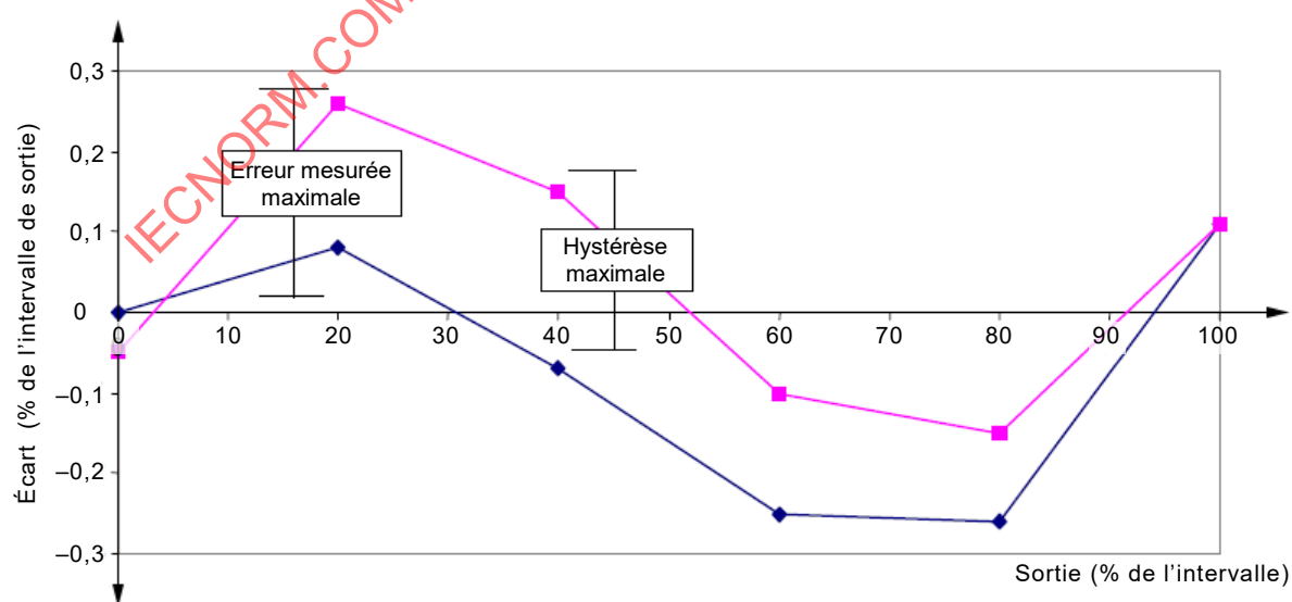
Figure 3 – Exemple de tracé d'erreur mesurée
