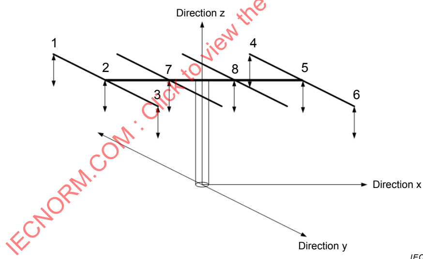
Figure 5 – Exemple d'emplacements de mesure de la déviation structurelle
