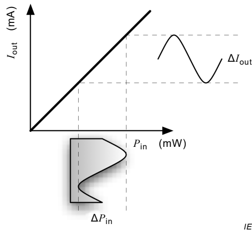
Figure 1 – Définition de "l'efficacité de conversion"
