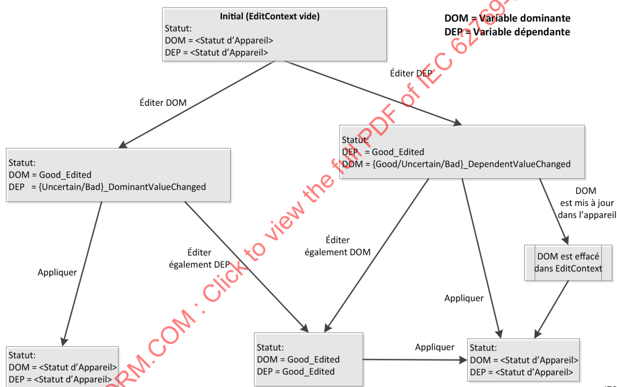
Figure 4 – Diagramme d'états EditContext Online pour les Variables dominantes et dépendantes
