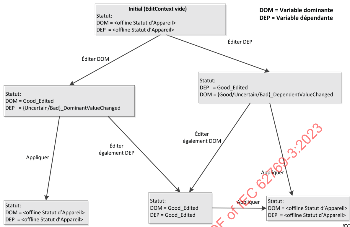
Figure 5 – Diagramme d'états EditContext Offline pour les Variables dominantes et dépendantes
