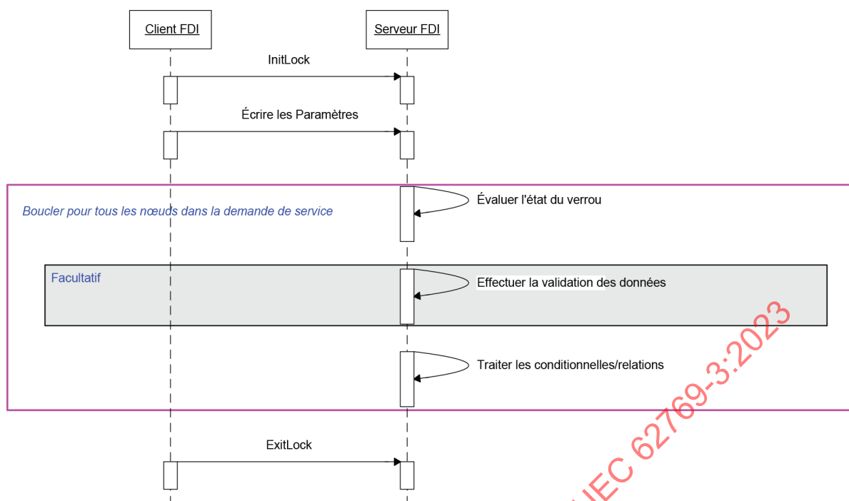
Figure 9 – Ecriture immédiate de variables hors-ligne
