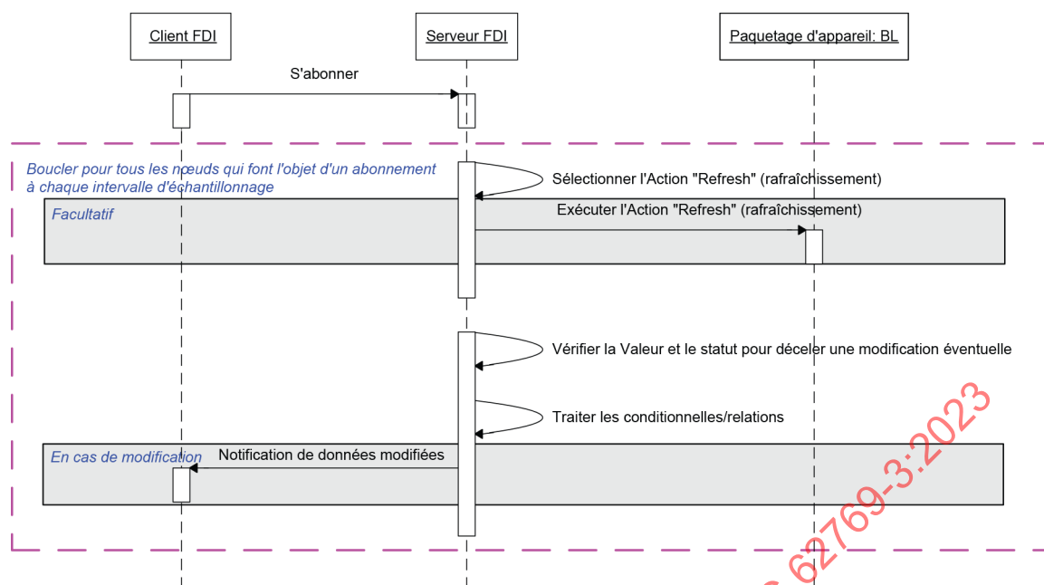
Figure 12 – Abonnement aux variables hors-ligne
