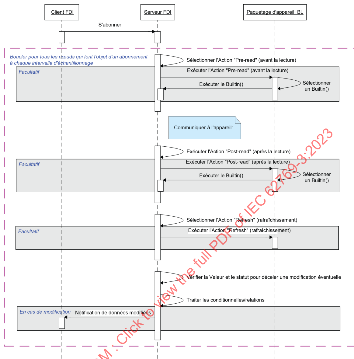
Figure 13 – Abonnement aux variables en ligne
