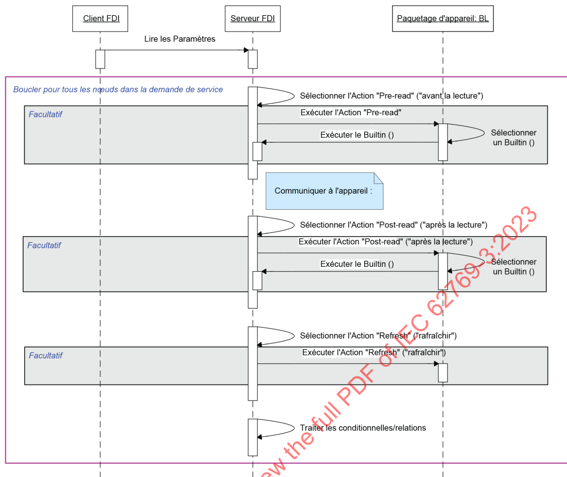
Figure 8 – Lecture de variables en ligne
