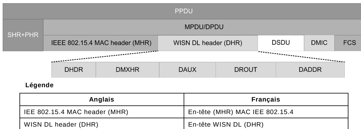
Figure 88 – Structure de PhPDU et de DPDU
