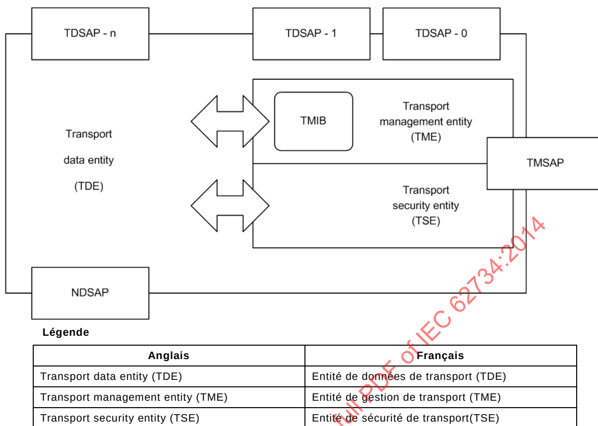
Figure 107 – Modèle de référence de TLE
