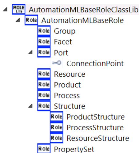
Figure 14 – Bibliothèque de classes de rôles de type AML
